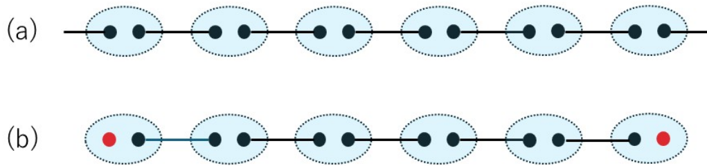
図 1 : (a) AKLT 状態の模式図。黒丸は S=1/2 のスピンを表し、楕円は二つの S=1/2 スピンの合成による S=1 スピンを示している。二つの黒丸を結ぶ実線はスピン一重項( S=0 )を表す。(b) 有限長の AKLT 状態の両端には S=1/2 のスピン (赤丸) が余っている。
