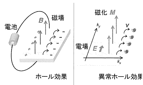
SrRuO 3 における異常ホール効果 - 運動量空間における磁気単極子
