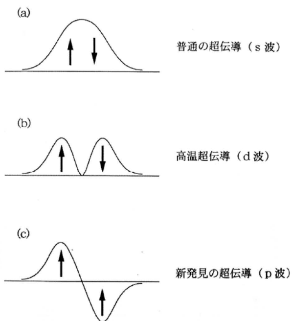
図4. 超伝導の電子対モデル (矢印はスピン)
