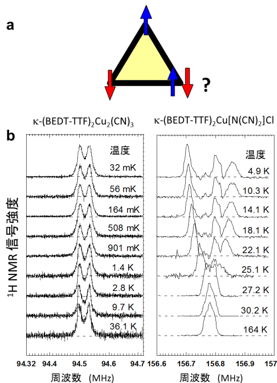
図 1 a 三角格子上の反強磁性スピン. b 三角格子物質（左図）と歪んだ三角格子物質（右図）の ^1\text{H} NMR 吸収線. 吸収線の温度変化の有無は磁気秩序の存否に対応する。
