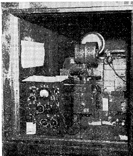
第5図 仁科式電離箱。
