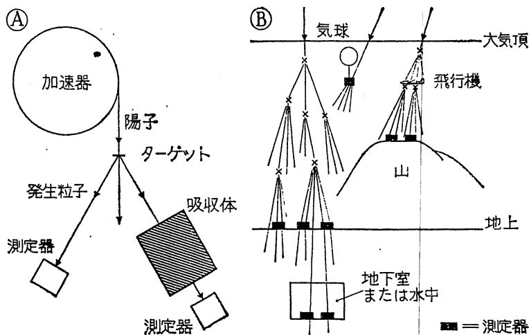
第8図 加速器と宇宙線測定器の基本的配置。
