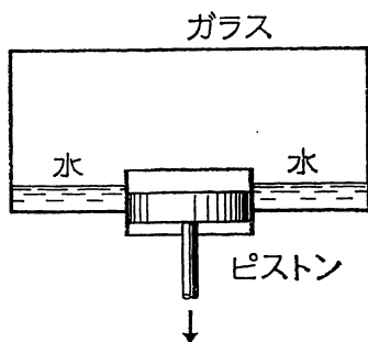
第6図 ウィルソン霧箱の原理。
