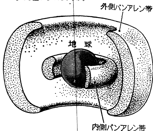
第9図 バンアレン帯。
