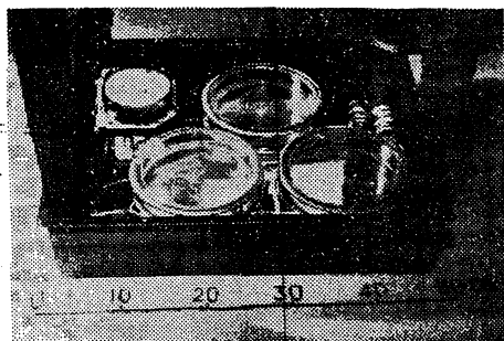
第7図 スパークチェンバー。
