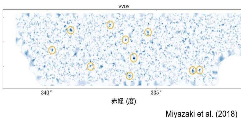
図2. 弱重力レンズ効果により求めた暗黒物質分布(青色)と同定された銀河団(黄色○)
