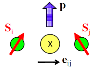
図2. 非共線的磁気構造が分極を誘起する機構。隣り合うスピン S_1 、 S_2 が互いに傾いた(非共線な)配置を取ると、スピン面に平行でかつ二つのスピンを結ぶベクトルに垂直な方向に電気分極 P が発生する。
