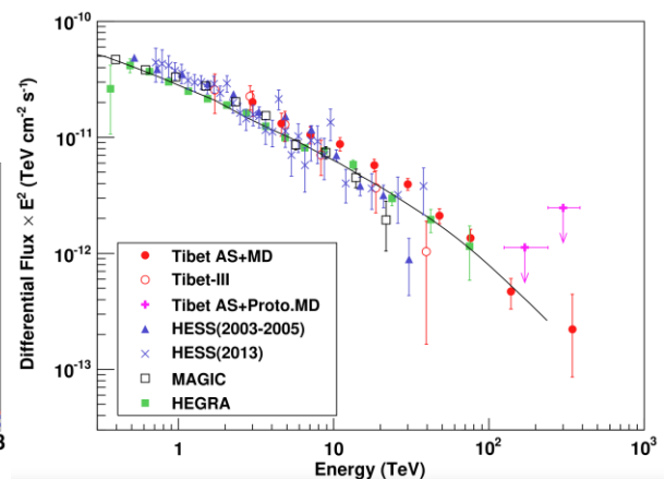
図3:左)Tibet AS \gamma 実験で観測された100TeV以上のガンマ線候補イベントの到来方向とかに星雲の方向との相関。右)かに星雲の方向からのガンマ線のエネルギースペクトル。初めて100TeVを超えるエネルギーのガンマ線が観測された。(文献[1]より)
