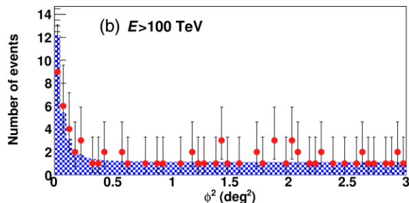
図3:左)Tibet AS \gamma 実験で観測された100TeV以上のガンマ線候補イベントの到来方向とかに星雲の方向との相関。右)かに星雲の方向からのガンマ線のエネルギースペクトル。初めて100TeVを超えるエネルギーのガンマ線が観測された。(文献[1]より)
