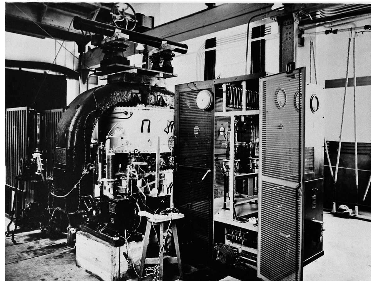
小サイクロトン全体写真 第3号はほぼ同じ形状
